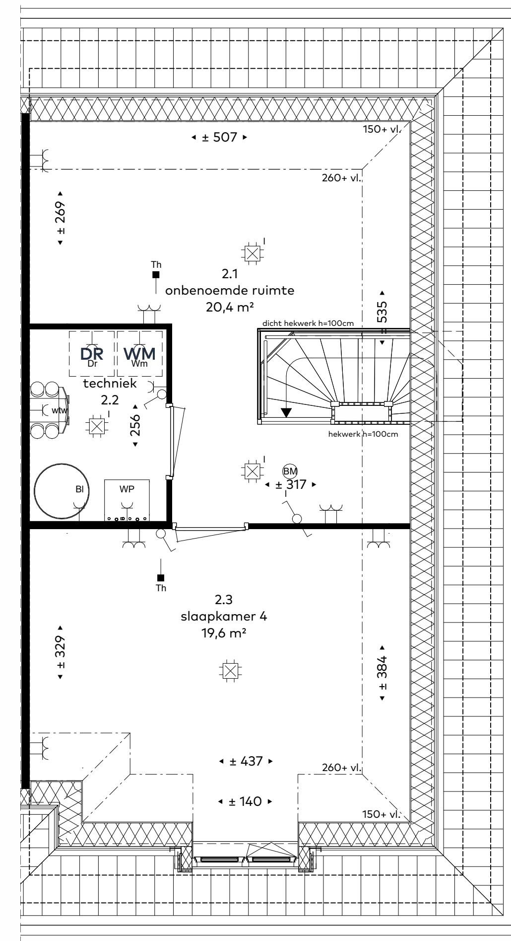
VB2 - tweede verdieping standaard
